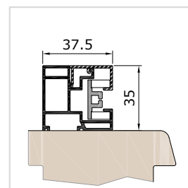
Führungsschiene FS Z37VP, Putzvariante
