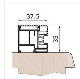
Standard Führungsschiene FS Z37VS
