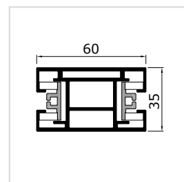
freitragende Kämpferschiene FS ZT60V
