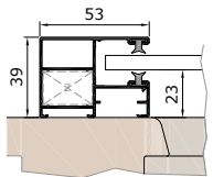
Führungsschiene KF53V
