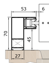
Führungsschiene ED53V
