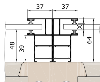
Kämpfer mit 2x Führungs- schiene KD37R /*GD37R
