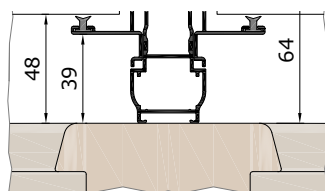
Kämpfer mit 2x Führungs- schiene KD37R /*GD37R
