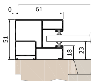
Führungsschiene KF61K
