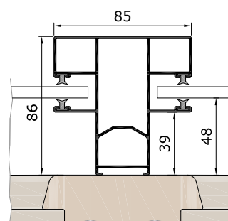
Führungsschiene KD85K
