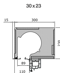
Kastengrößen [mm]
