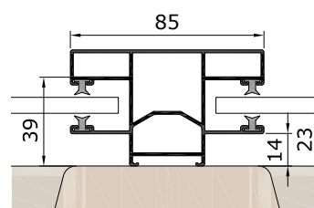
Führungsschiene KE85K
