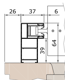
Führungsschiene FD37R
