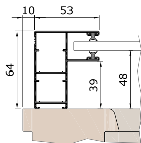
Führungsschiene KD53R /*GD53R
