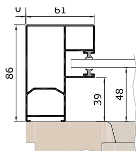
Führungsschiene KD61K
