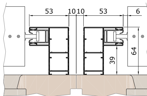
2x Führungsschiene mit FD53R
