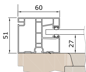
Führungsschiene K60AE
